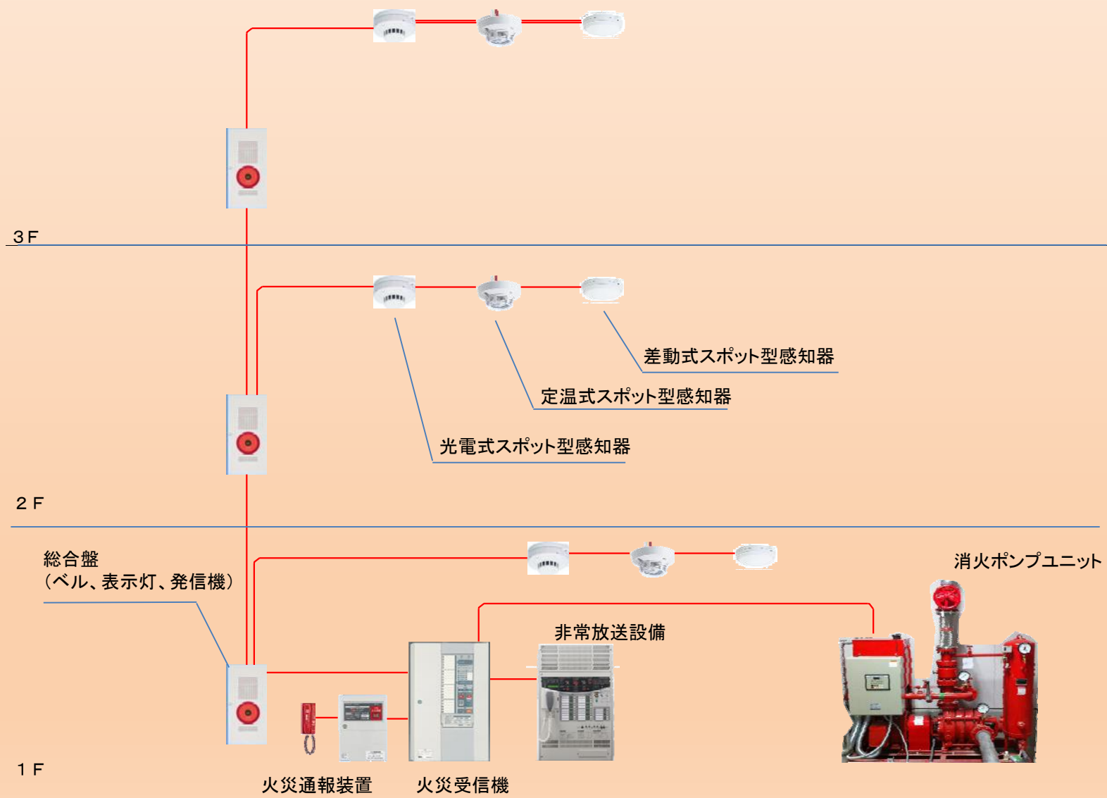
<自動火災報知設備 構成例>
